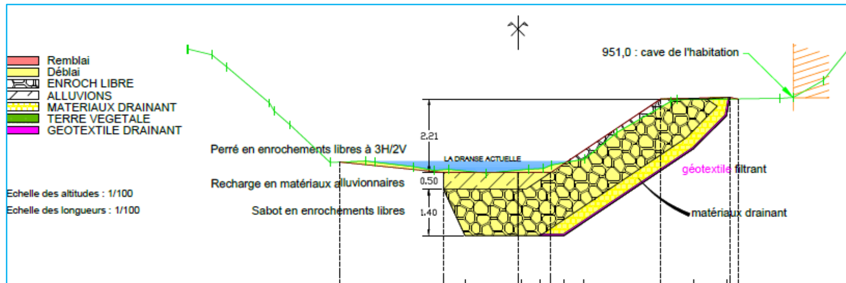
Les Ogays – coupe de principe de la protection de berges
