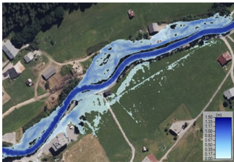
Le Malève – modélisation crue Q10
